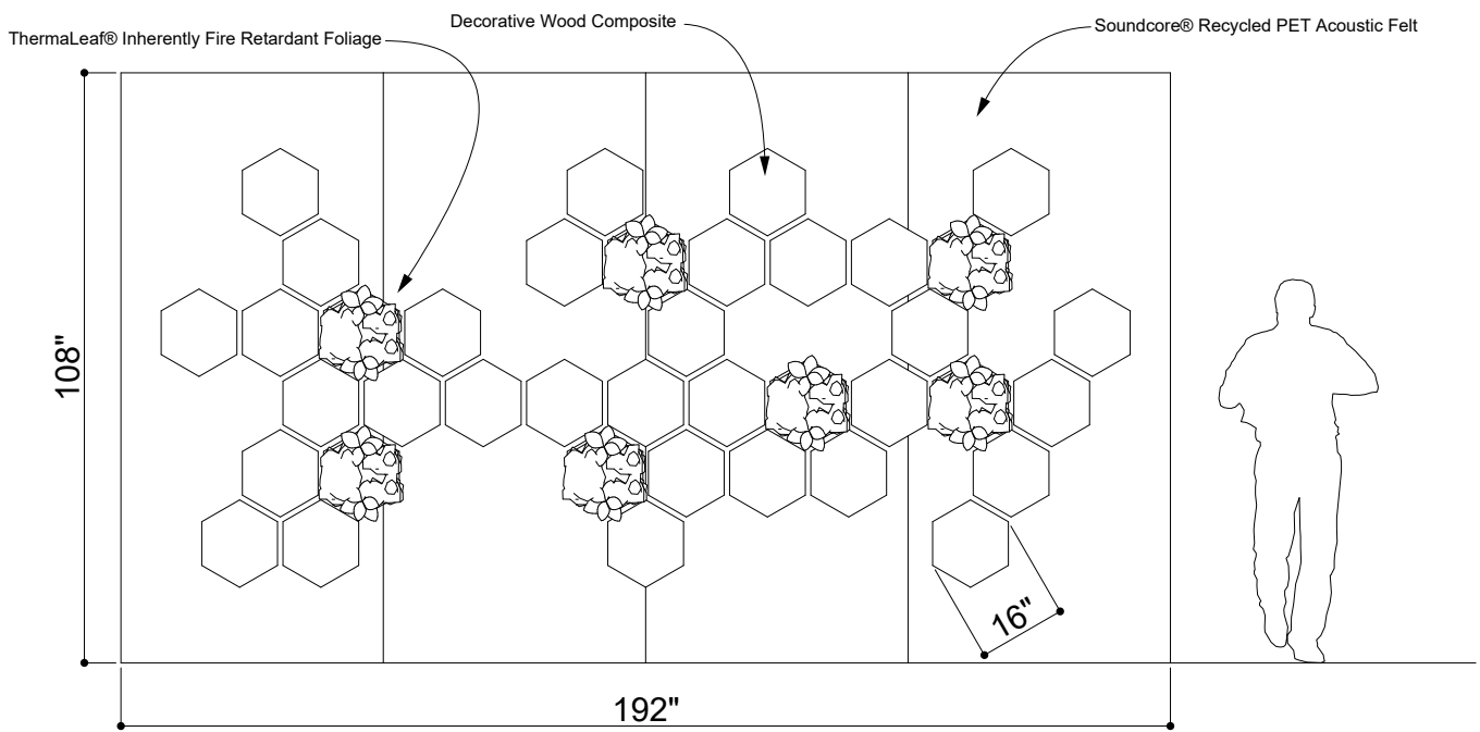
① ELEVATION 1
